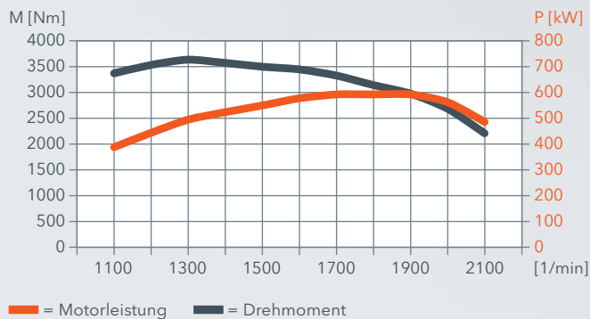
Motorkennlinien Kaltfräse W 220 Fi
